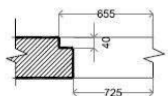
SEZIONE G-G
